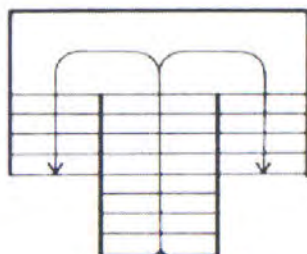
踊場付き両返し階段
